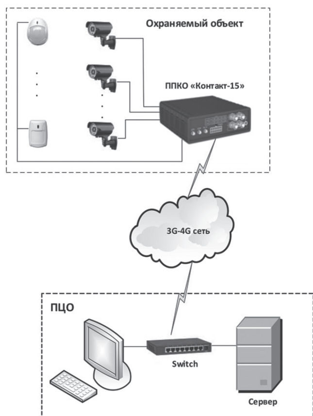
Рис. 2. Схема построения видеоподсистемы в составе системы мониторинга «Контакт» с применением охранного прибора «Контакт-15»
