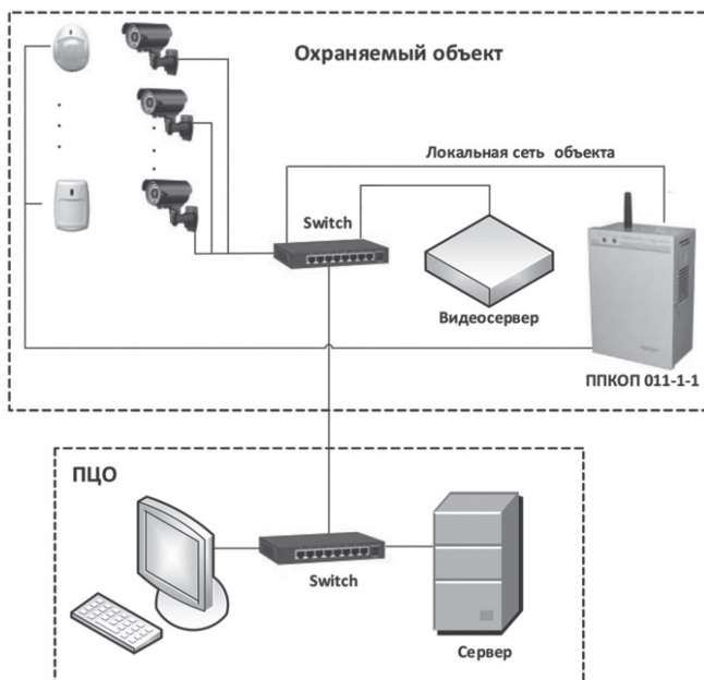
Рис. 1. Схема построения видеоподсистемы в составе АСЦН «Приток-А» с применением оборудования Domination
