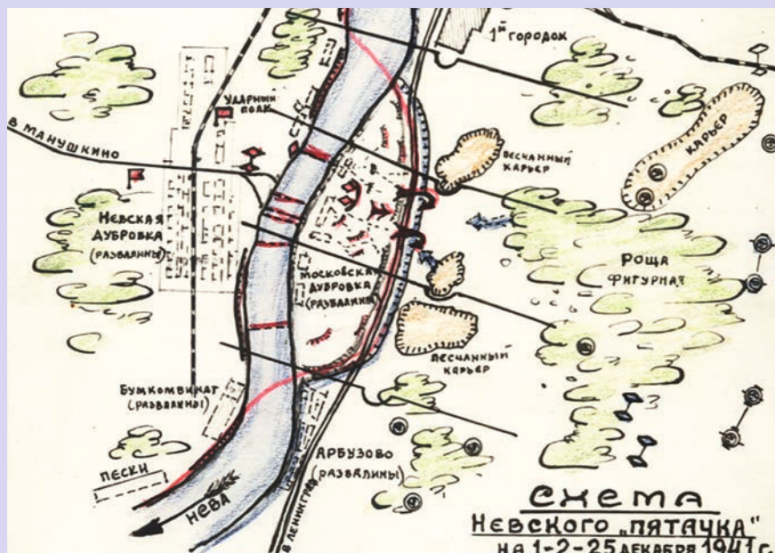
Схема «Невского пятачка», декабрь 1941 г.
