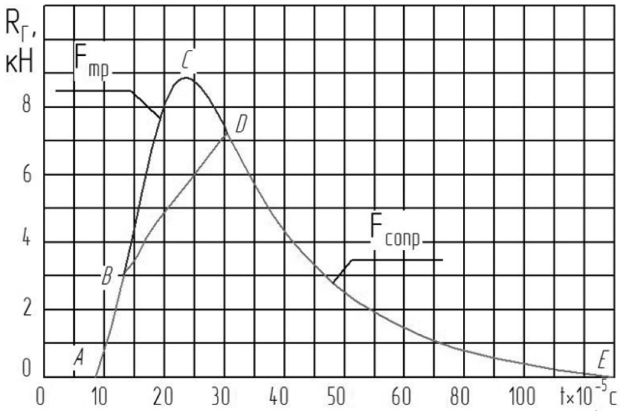
Рис. 3. Изменение силы сопротивления при заклинивании гильзы и отсутствии периода заклинивания
