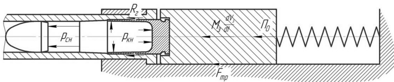
Рис. 2. Расчетная схема систем с инерционным запиранием, где
