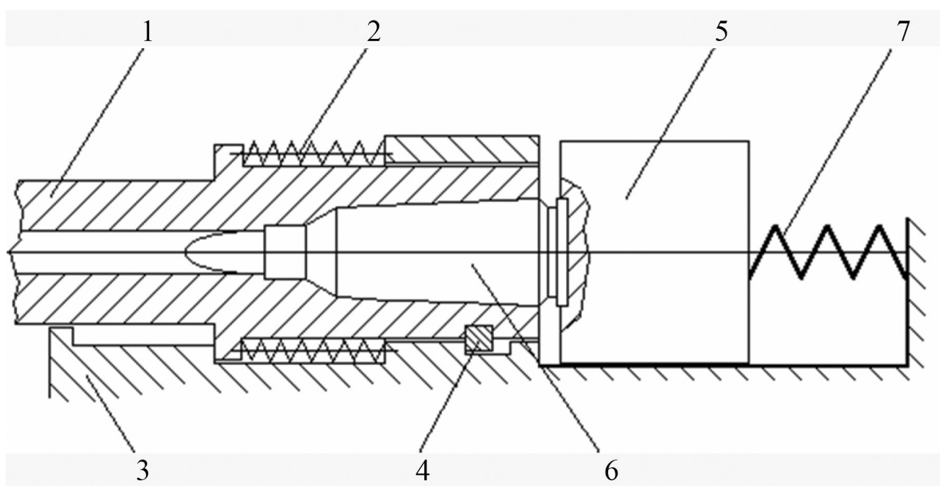
Рис. 4. Конструктивная схема автоматики со свободным затвором и подвижным стволом: 1 – ствол; 2 – пружина ствола; 3 – ствольная коробка; 4 – шпонка ствола; 5 – свободный затвор; 6 – патрон; 7 – возвратная пружина
