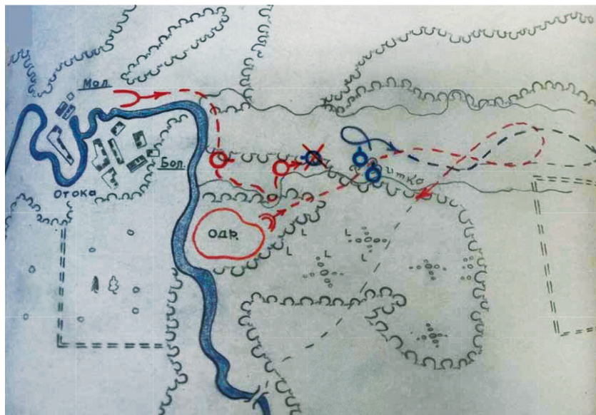
Рисунок 7. Схема действий наряда 3-й роты 137-го сп по преследованию и задержанию группы дезертиров 22 июня 1942 г.
