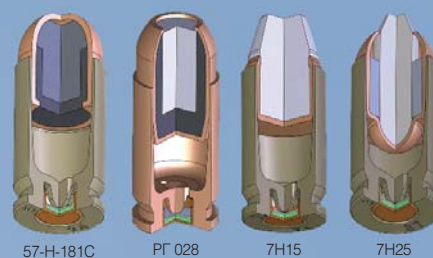
Схемы некоторых 9-мм патронов, используемых для стрельбы из АЕК-919К «Каштан»
