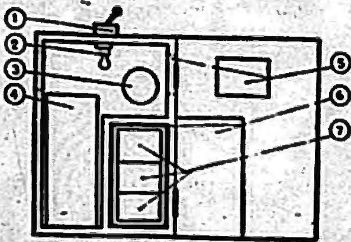
Чертеж 3. Расположение узлов в ящике: 1 — выключатель; 2 — патрон с лампочкой; 3 — звонок; 4 — прибор «Яттарь»; 5 — окно; 6 — проводка со стороны; 7 — три элемента Зс.
