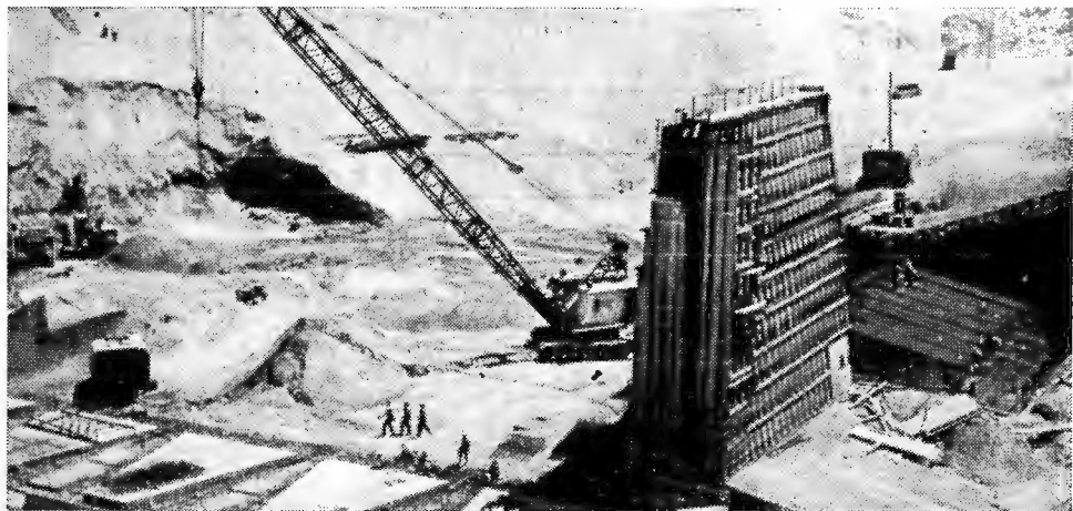
Строительство шестой насосной станции на канале.
