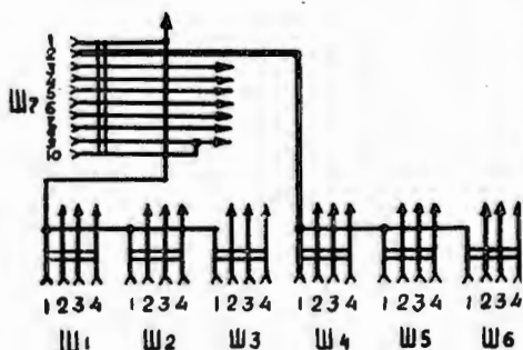
Рис. 2. Принципиальная электрическая схема распределительной коробки РК-М после переделки.
