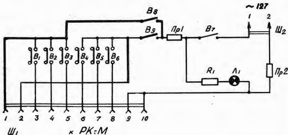
Рис. 1. Принципиальная электрическая схема универсального пульта управления (УПУ-М).
