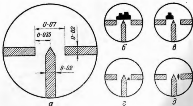
Рис. 2. Определение расстояний с помощью оптического прицела.
