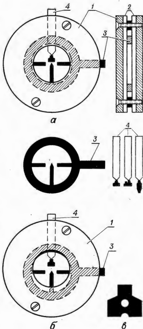
Рис. 1. Показная снайперская мушка.
