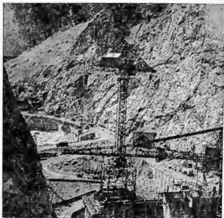
На реке Нарын в Киргизии возводится Токтогульская ГЭС мощностью один миллион 200 тысяч киловатт. Это первая в практике гидростроительства высотная электростанция в сейсмическом районе.
