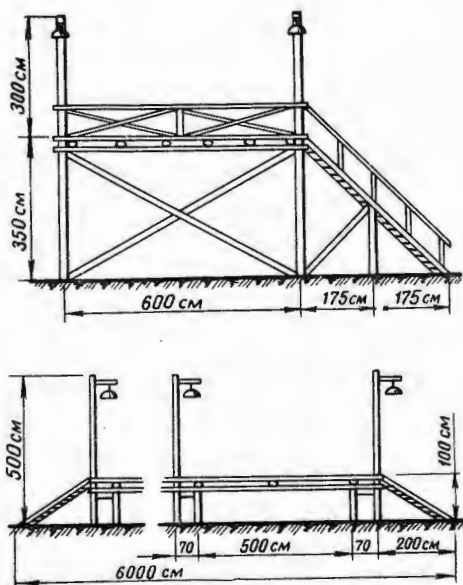
Рис. 1. Площадка и трап (внизу) для осмотра вагонов (вариант).
