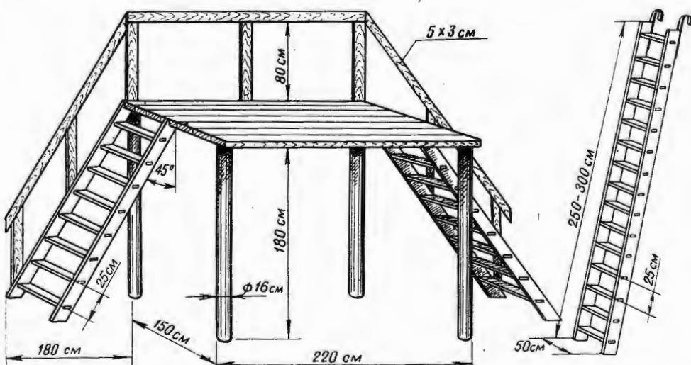
Рис. 2. Площадка и лестница (справа) для осмотра автотранспорта (вариант).
