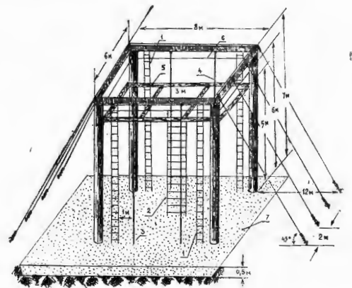
Рис. 2. Схема металлической [деревянной] прямоугольной конструкции: 1 — вертикальная лестница, 2 — вертикальный лабиринт, 3 — шест, 4 — канат, 5 — горизонтальная опора, 6 — леер для страховки, 7 — яма с опилками глубиной 0,5 м, 8 — тренажер для метания гранат.
