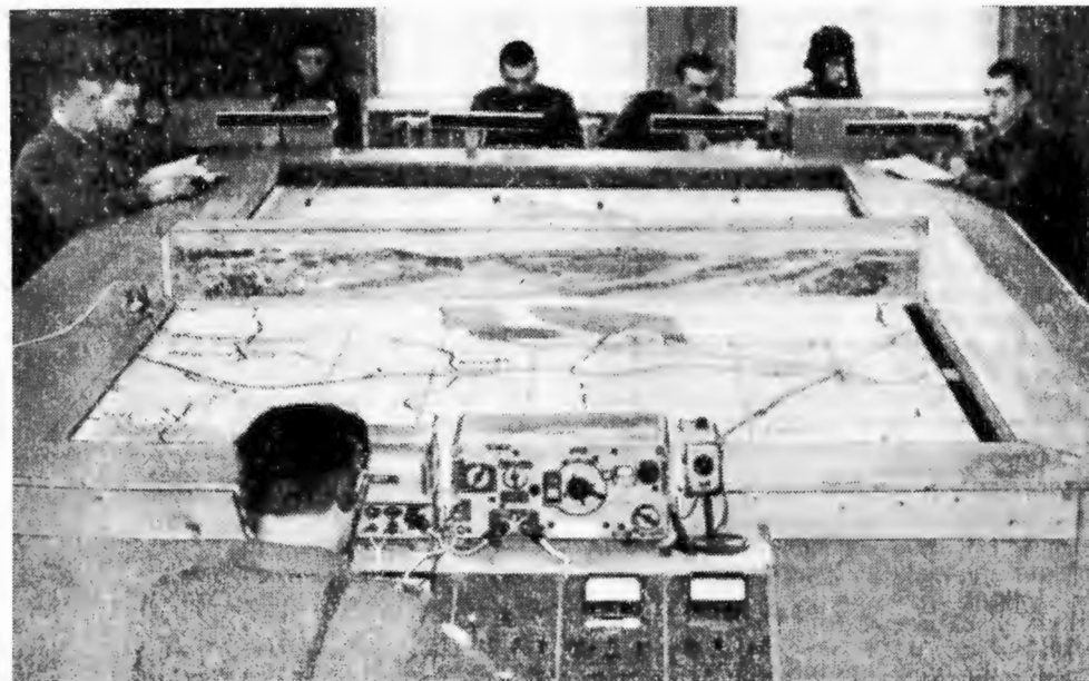
На снимке: общий вид тренажера для подготовки химиков-разведчиков. Занятие проводит старший лейтенант В. Думнов.
