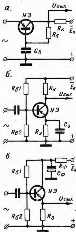
Рис. 1. Однокаскадные усилители.
