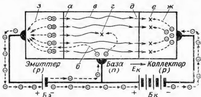
Рис. 2. Схема распределения тока эмиттера в транзисторе типа p-n-p .
