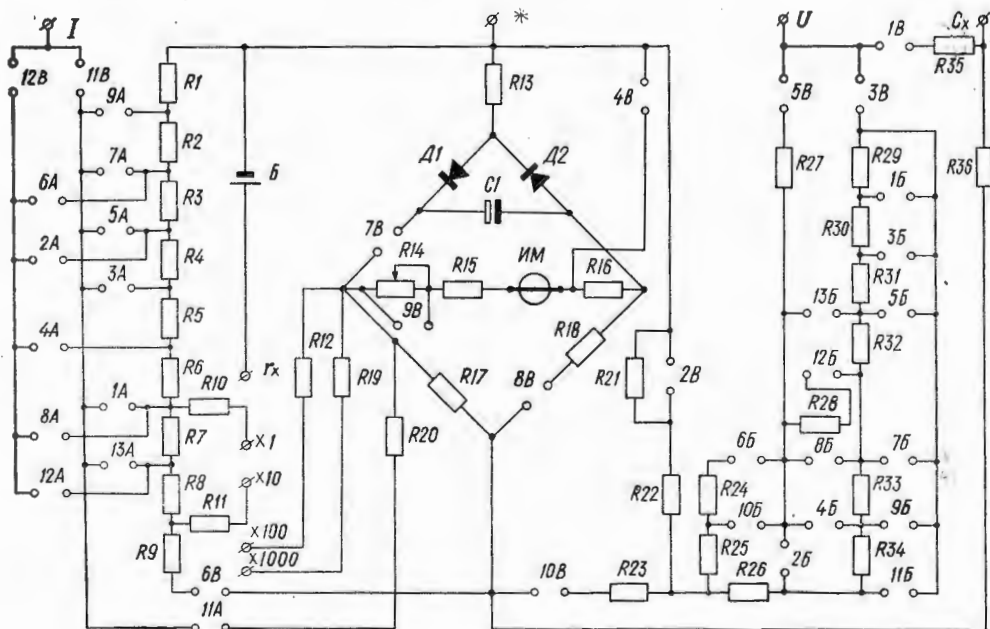
Рис. 2. Принципиальная схема прибора и таблицы замыканий контактов переключателей.
