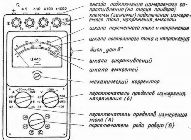
Рис. 1. Внешний вид прибора Ц435.
