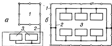
Рис. 2. Схемы выносного [а] и контурного [б] заземления. 1 — заземлитель; 2 — заземляющие проводники [магистраль]; 3 — заземляемое оборудование.
