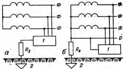
Рис. 1. Принципиальные схемы защитного заземления и металлического соединения корпусов электроустановок с нулевым проводом.
