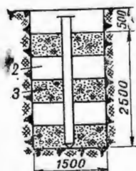
Рис. 4. Заземлитель с местной обработкой земли: 1 — заземлитель; 2 — поваренная соль; 3 — грунт.
