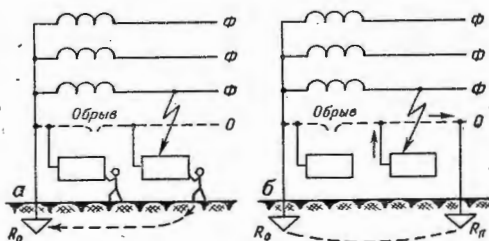
Рис. 5. Схемы протекания тока при обрыве нулевого провода: а — при отсутствии повторного заземления; б — при наличии повторного заземления.
