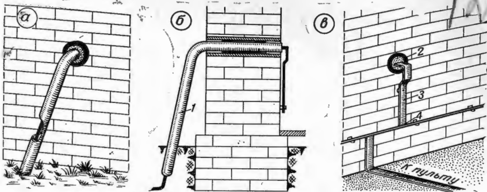
Рис. 3. Ввод заземлительной полосы в здание.
