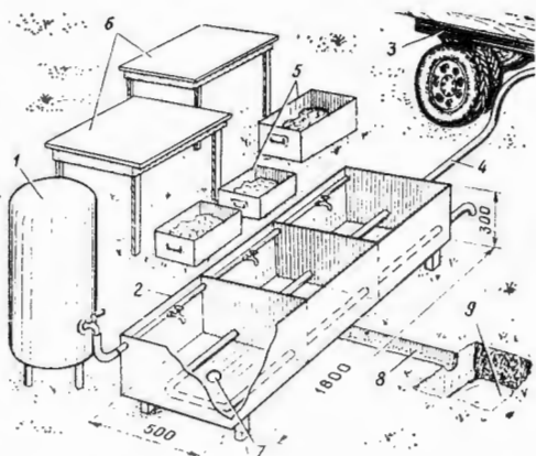
Схема места расконсервации котелков
