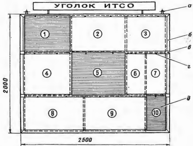
Рис. 1. Стеллаж технического уголка: а — прошина; б — каркас; в — горизонтальная рейка; г — штырь для планшетов; д — планшет.
