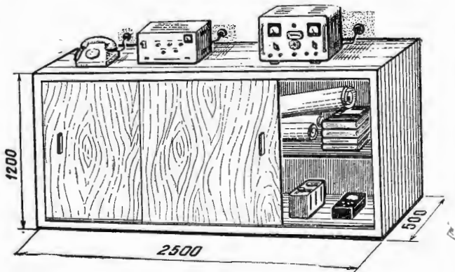
Рис. 2. Стеллаж технического уголка.
