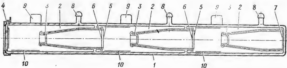
Рис. 2. Электронно-оптический преобразователь (ЭОП):
