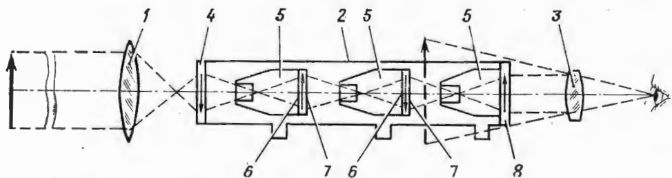
Рис. 1. Принципиальная схема построения изображения ночным бесподсветным прицелом:
