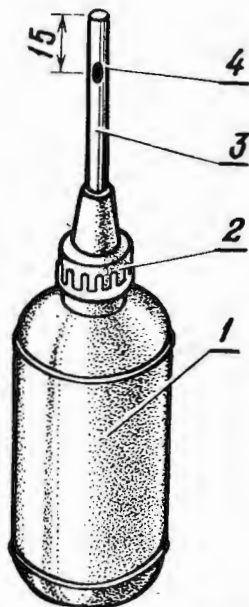
Рис. 3. Баллон для ручной доливки воды.
