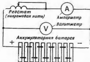
Рис. 2. Схема разряда аккумуляторных батарей.
