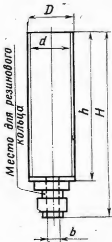
Рис. 1. Защитная трубка.
