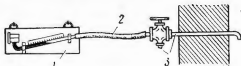
Рис. 2. Схема установки подпоромера: 1) подпоромер; 2) резиновый шланг; 3) трубка с газовым краном.
