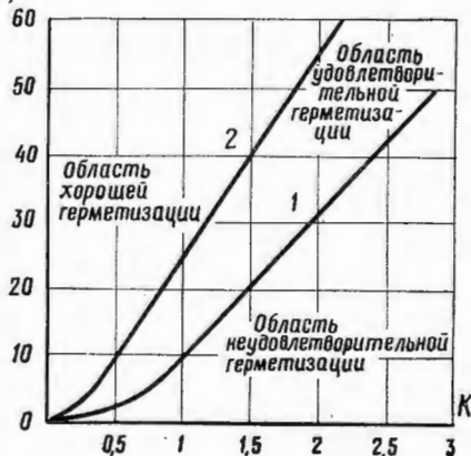
Рис. 3. График оценки герметичности убежищ:
