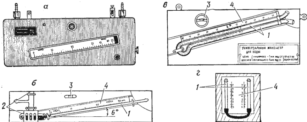
Рис. 1. Приборы для определения подпора воздуха в убежище: а) тягонапомер ТНЖ; б) наклонный манометр; в) универсальный манометр (подпоромер КГ); г) простейший манометр (1 — стеклянные трубки; 2 — стеклянный резервуар с соском для наливания жидкости; 3 — уровень; 4 — подвижная шкала).
