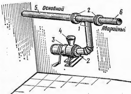
Рис. 4. Переносная установка для проверки на герметичность убежища, не имеющего ФВА:
