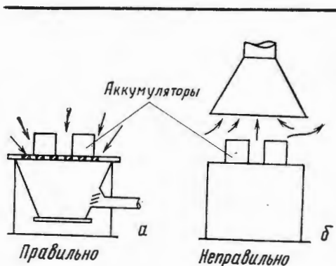
Рис. 2. Схема местного отсоса.
