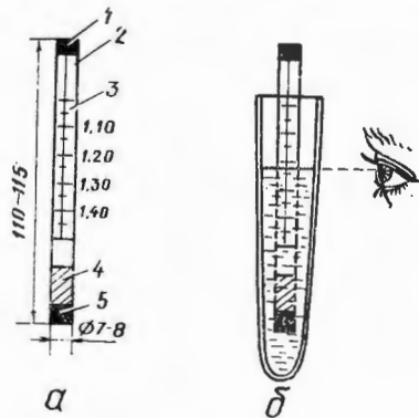
Рис. 1. а — самодельный ареометр, б — порядок пользования.
