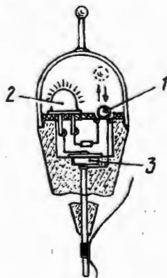
Конструкция светящегося поплавка
