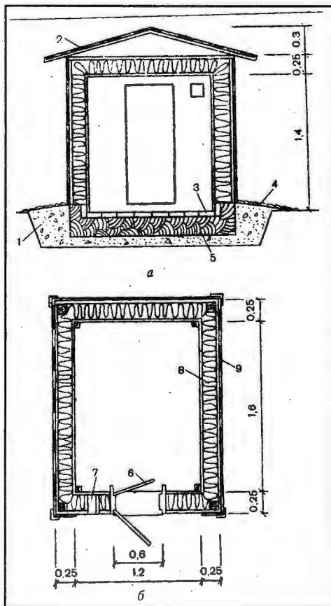
Схема мини-погреба (а—разрез, б—план): — песчано-щебеночная подготовка, 2 — двускатная кровля, 3 — кирпичный пол, 4 — отмостка, 5 — глиняный замок, 6 — дверь, 7 — вентиляционное окно, 8 — утеплитель, 9 — гидроизоляция.
