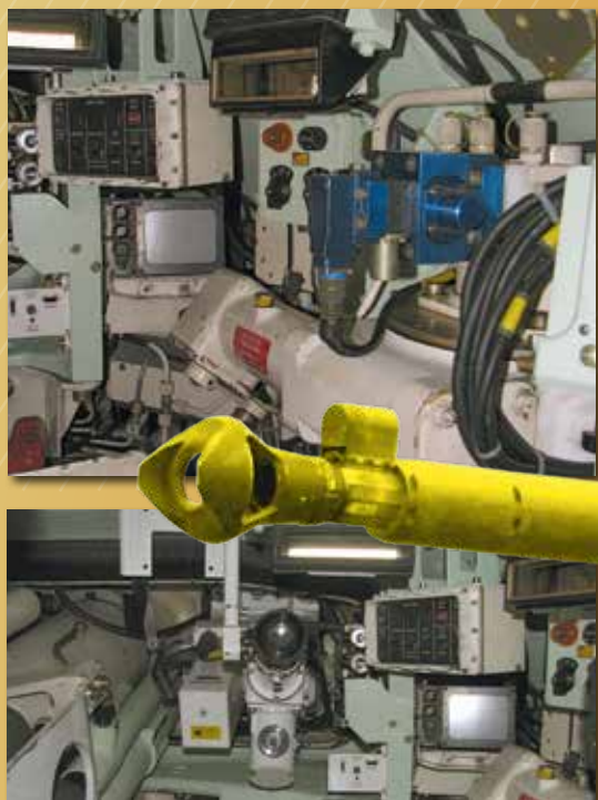
Место командира (вверху) и наводчика (вид изнутри)
